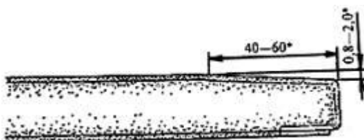
Рисунок 2 - Утоненная с лицевой стороны кромка (УК)
