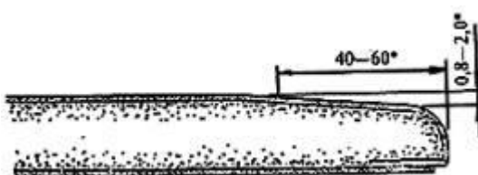
Рисунок 4 - Полукруглая и утоненная с лицевой стороны кромка (ПЛУК)
